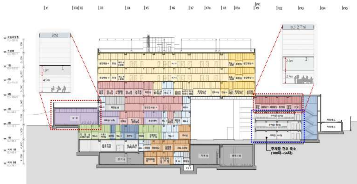
< 단면도 >
